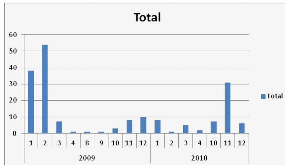
Fig. 1 : distribution mensuelle des observations de Goéland à bec cerclé en Aquitaine en 2009 et 2010
