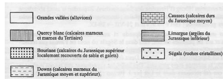
Carte géomorphologique du Lot
