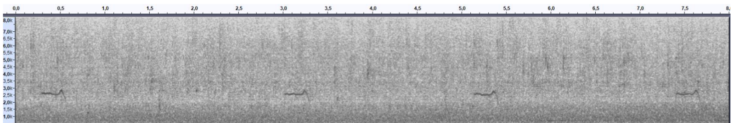
Fig. 46 : Grand Gravelot, nuit du 25 au 26 août 2023, Thorigny-sur-Marne-77 (JB). XC827362
